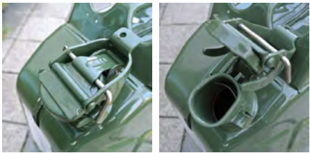
Taniche in acciaio resistente ai raggi U.V. con trattamento anticorrosivo interno e verniciatura epossidica esterna. Tappo in metallo inamovibile con chiusura progressiva e totale ad incastro. Steel tanks resistant to UV rays with with internal anticorrosive treatment and epoxy painting outside. Metal cap immovable with progressive closing and total interlocking.
